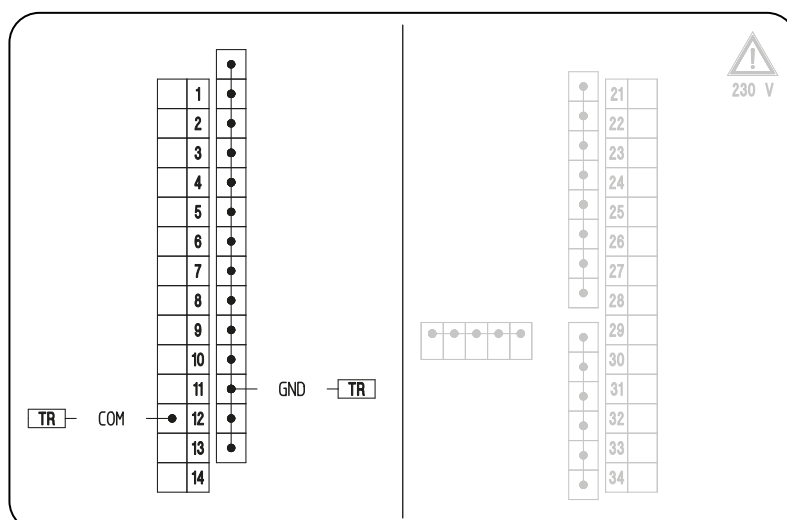
Illustration.2 - Schéma des connexions de la régulation, côté basse tension
