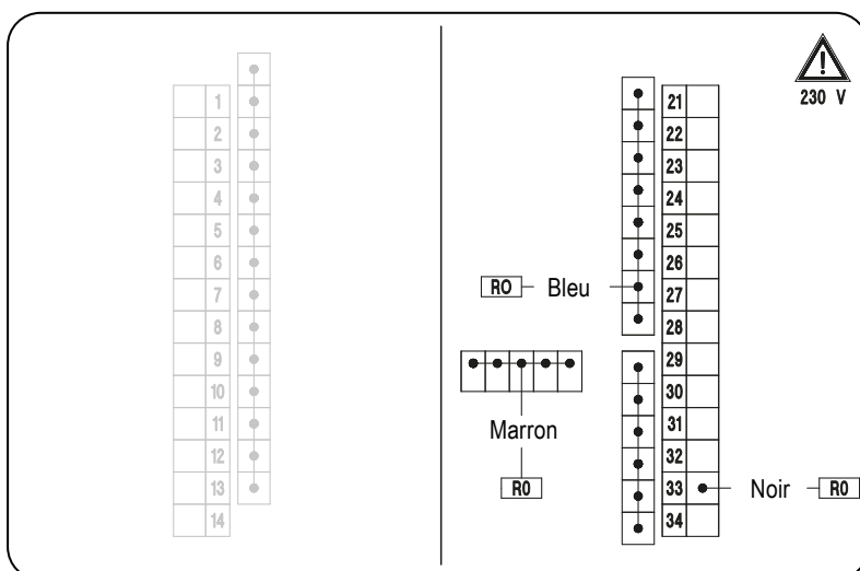
Illustration.3 - Schéma des connexions de la régulation, côté 230V
